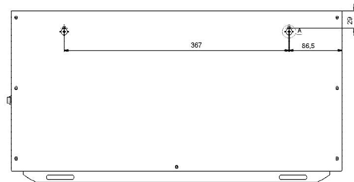
Габаритные и установочные размеры стабилизатора напряжения переменного тока LIDER PS10000SQ-15
