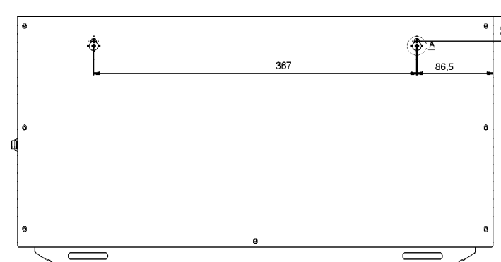
Габаритные и установочные размеры стабилизатора напряжения переменного тока LIDER PS12000SQ-15
