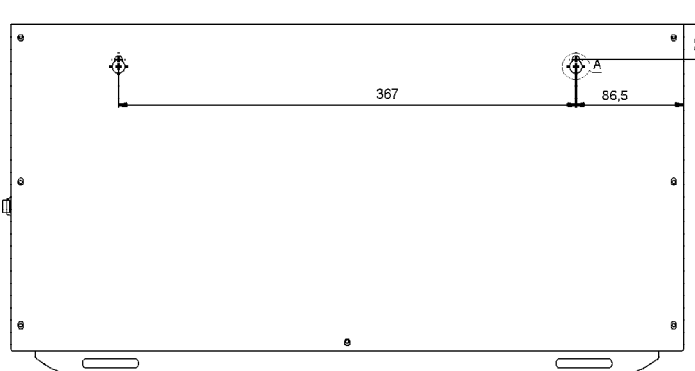
Габаритные и установочные размеры стабилизатора напряжения переменного тока LIDER PS3000SQ-25
