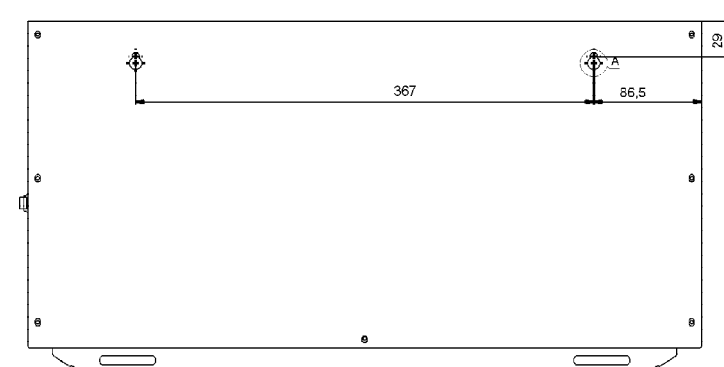
Габаритные и установочные размеры стабилизатора напряжения переменного тока LIDER PS7500SQ-25
