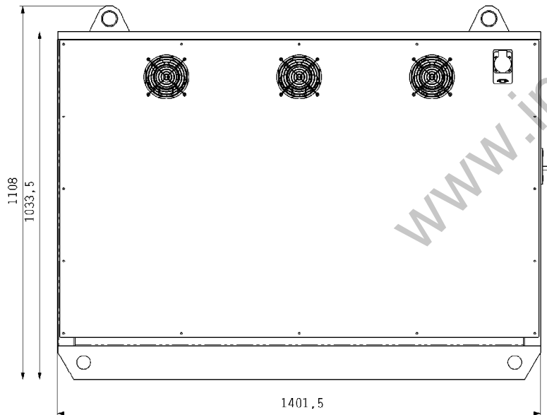
Габаритные и установочные размеры стабилизаторов напряжения переменного тока LIDER PS100000SQ-IM-15
