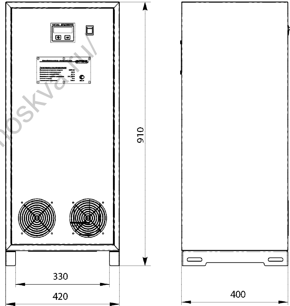
Габаритные и установочные размеры стабилизаторов напряжения переменного тока LIDER PS12000SQ-I-25
