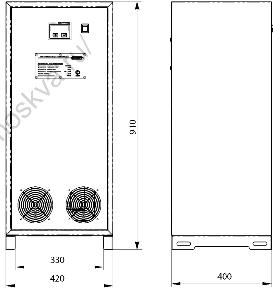
Габаритные и установочные размеры стабилизаторов напряжения переменного тока LIDER PS7500SQ-I-40
