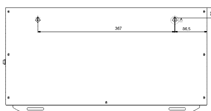
Габаритные и установочные размеры стабилизатора напряжения переменного тока LIDER PS12000W-30
