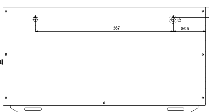
Габаритные и установочные размеры стабилизатора напряжения переменного тока LIDER PS3000W-30
