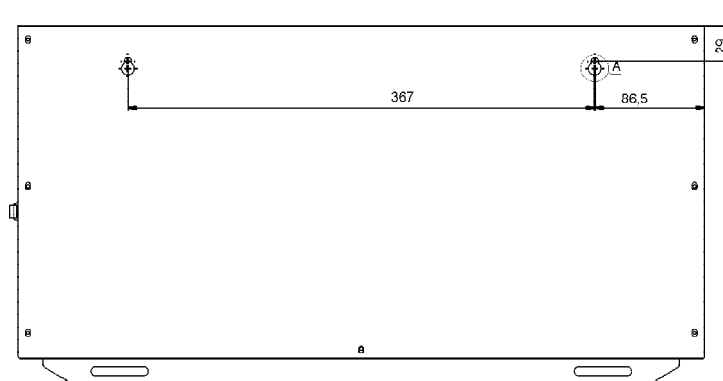
Габаритные и установочные размеры стабилизатора напряжения переменного тока LIDER PS7500W-50
