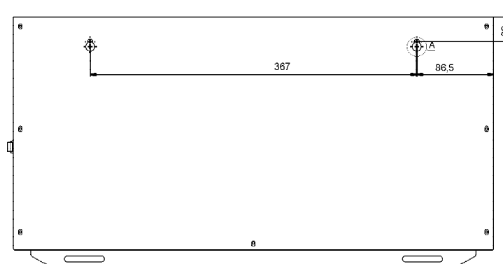
Габаритные и установочные размеры стабилизатора напряжения переменного тока LIDER PS7500W-SD
